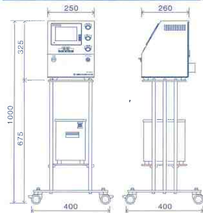
自立専用台 取付寸法(キャスター付)
