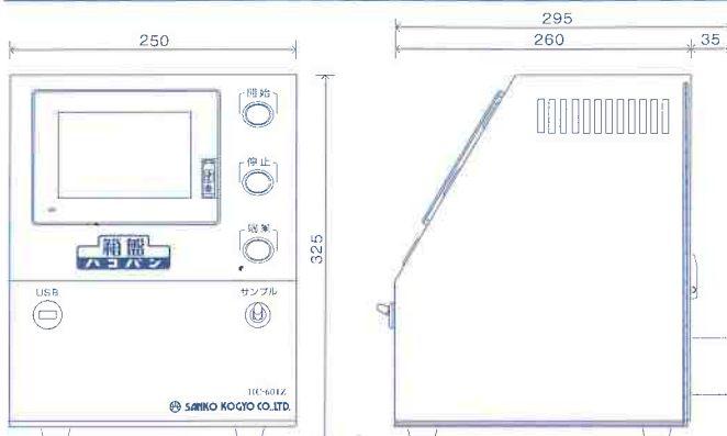
箱盤 外形寸法
